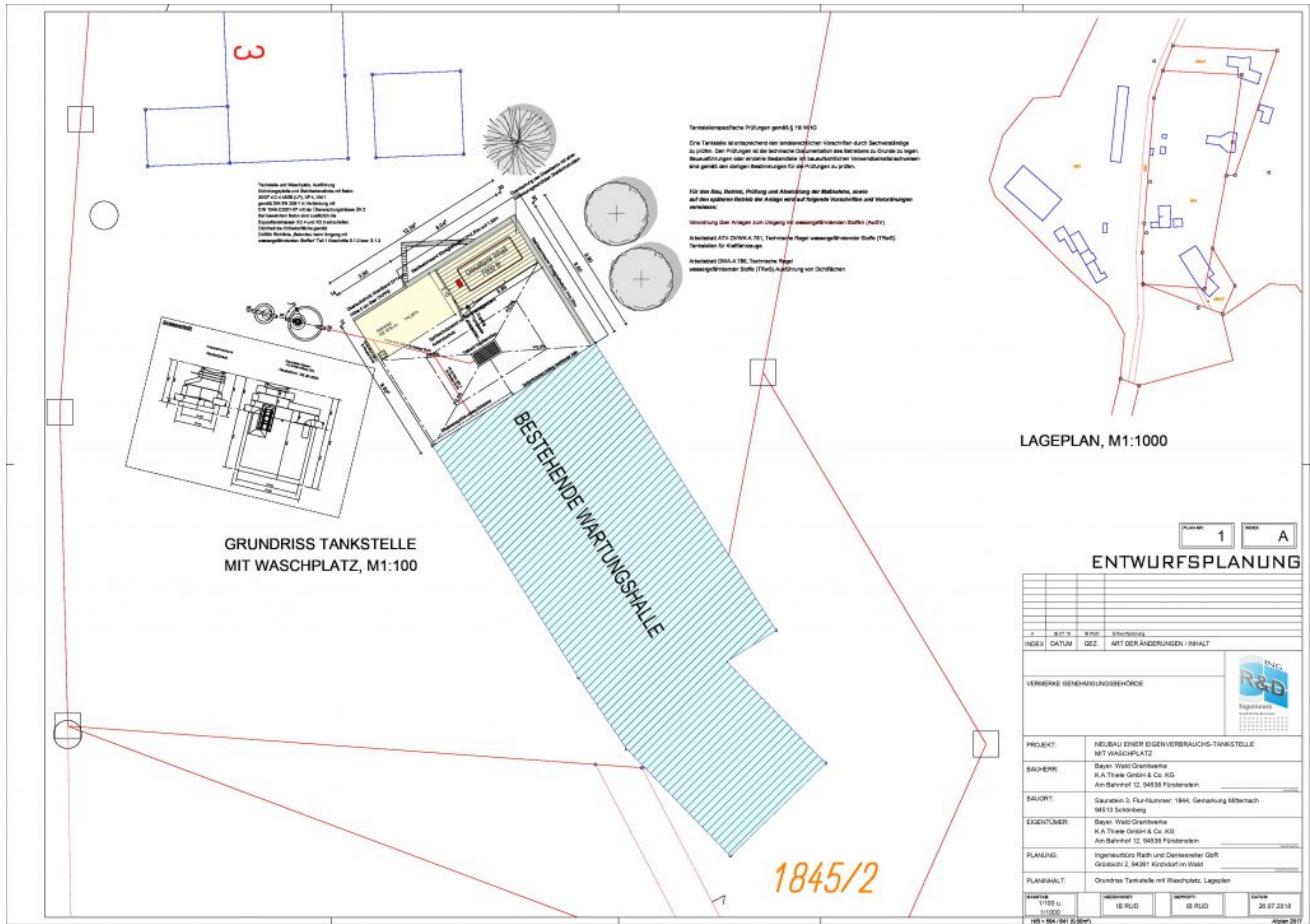
Planung einer neuen Tankstellenanlage
